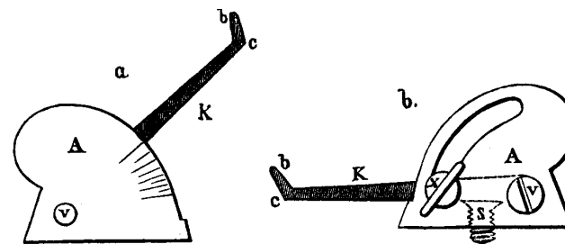
Fig. 18 a und b. Schweizer Visier. A Visierbacken. K Klappe. b c Kröpfung (in die Kimme eingeschnitten ist). x Druckschraube zum Feststellen der Visierklappe. v Visierschraube, um die sich die Klappe dreht. S Schraube zum Befestigen des Visiers auf dem Visierfuße.
