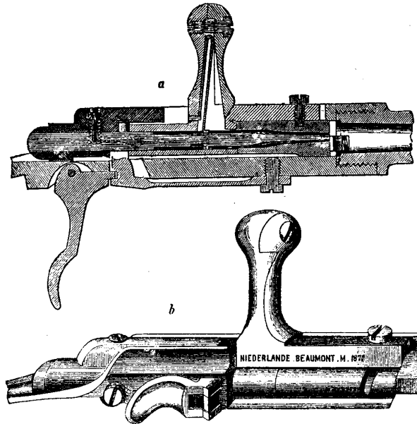
Fig. 54 a und b. Das System Beaumont. a Längsschnitt. b Ansicht von rechts. a Teilweise gespannt, weil der Hebelgriff mit Schlagfeder aufgestellt ist. b Entsiehert, weil Daumengriff rechts zurückgelegt ist.
