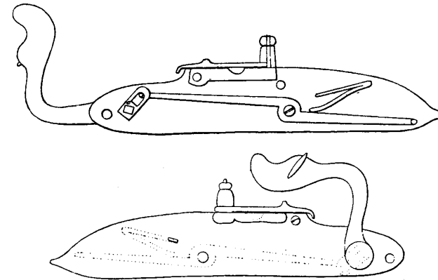
Fig. 2 a und b. Luntenschloß. Äußere und innere Ansicht.
