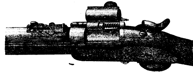
Fig. 46. Das System Snider. Verschuß zum Laden geöffnet.
