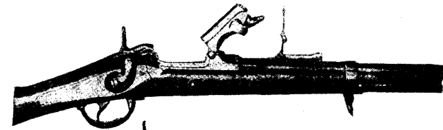
Fig. 49. System Terssen. Verschuß des belgischen Järgergewehrs von 1867. Geöffnet. Visierblatt des Leiter-Treppensichters aufgestellt.
