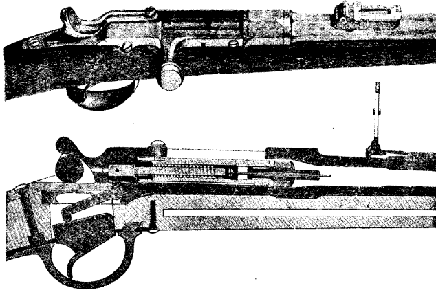
Fig. 39 a und b. Das französische Gewehr von 1865. System Chassepot.
