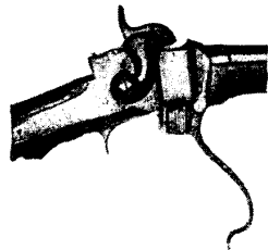
Fig. 34. System Sharps. Verschuß geöffnet. Das Zündplättchenmagazin geöffnet.
