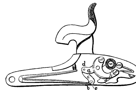
Fig. 13. Kettenschloß.
