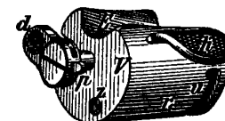
Fig. 45 b. Verschußstück. V Verschußblock mit p Verschußachse und d Verschußschraubenloch, sowie E Patroneneinlage. h Griff. u Ausziehernut. Z Zündstift. r 1 Zündstiftbegrenzungsschraube.
