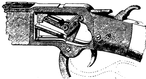
Fig. 59 a. Das System Henry & Winchester.
