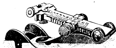
Fig. 69 b. Visier des englischen Gewehrs, 1903.
