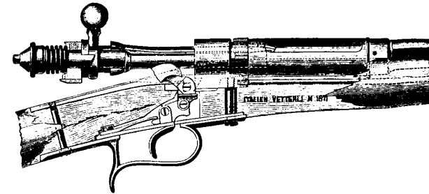
Fig. 52. Das System Vetterli. Verschluß geöffnet, Schloß gespannt, ohne Federgehäuse.
