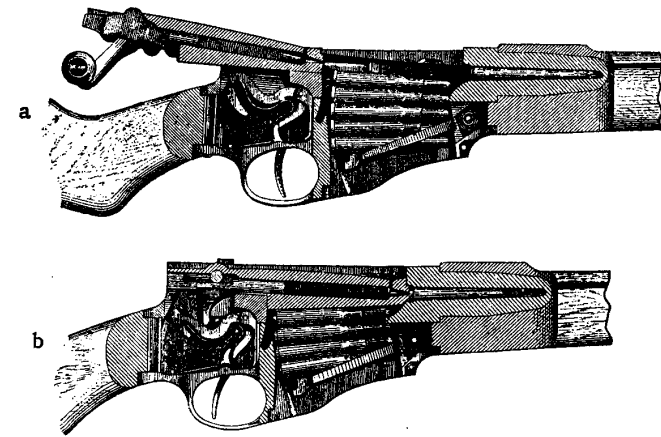
Fig. 65 a und b. Festes Lee-Magazin. Längsschnitt des nordamerikanischen Marine-Mehrladers von 1895. a Verschuß geöffnet. b Erste Patrone abgefeuert.
