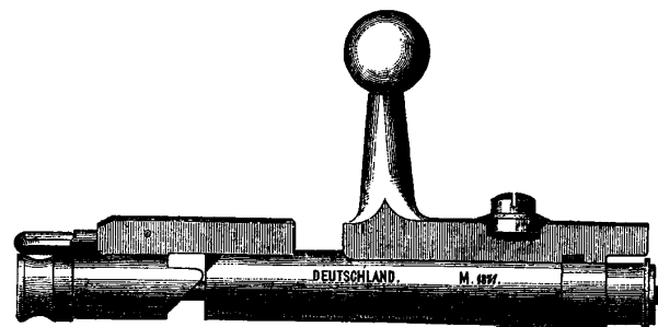
Fig. 53. Das System Mauser. Verschluss geschlossen, Schloß abgedrückt.
