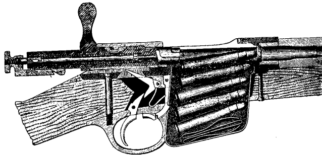
Fig. 64 b. Das System Lee (1879). h ist der Magazinhalter mit Daumengriff.
