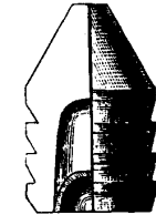
Fig. 26. Minié-Geschöß. Halb aufgeschnitten.
