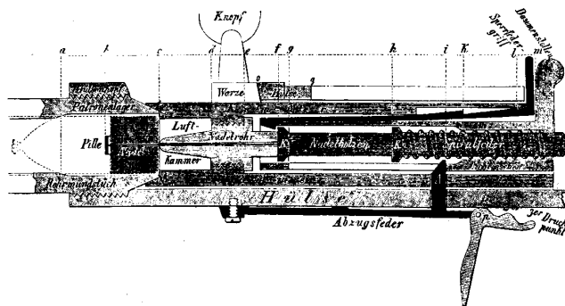
Fig. 38 b. Schloß des Zündnadelgewehrs. Schematische Darstellung.
