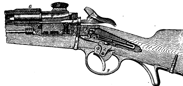
Fig. 45 a. Das System Werndl. Längsschnitt. Verschuß geöffnet. G Verschußgehäuse. P Auszieher. A Verschußachse. B Stoßplatte. V Verschußstück mit E Patroneneinlage und h Griff. d Verschußfeder. r Verschußfederschraube.
