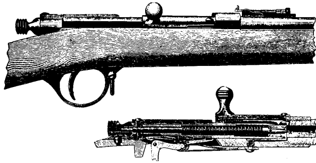
Fig. 55 a und b. Das System Berdan II. a Geschlossen und gespannt, Ansicht von der rechten Seite. b Längsschnitt, Griff zum Öffnen und Spannen aufgestellt.
