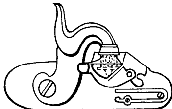
Fig. 15 b. Zünderschloß, Konstruktion Augustin 1842, geschlossen.
