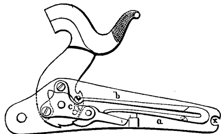
Fig. 14. Rückschloß.
