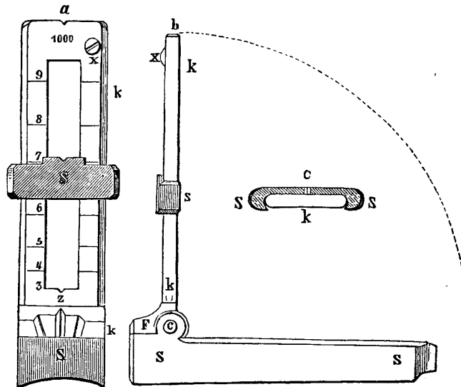
Fig. 19 a, b und c. Leiter-Schiebervisier.
