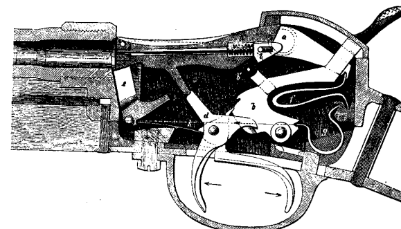
Fig. 42. Das System Werder.
