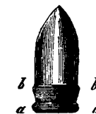
Fig. 23. Schweizerisches Spitzgeschoß von 1851 ohne Pflaster. a a und b b die Reibungsstellen des Geschosses im Laufe.
