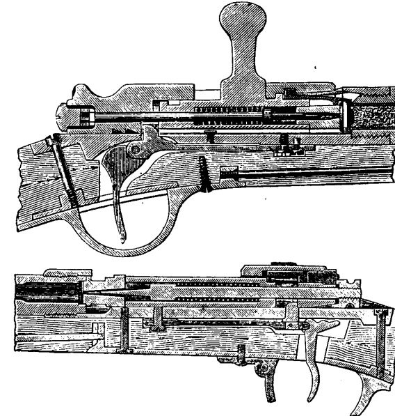
Fig. 56 a und b. Das System Gras. a Längsschnitt, Verschluss noch nicht völlig geschlossen und gespannt. b Längsschnitt, Verschluss geschlossen, abgefeuert.
