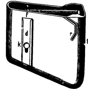
Fig. 64 a. Lee-Magazin. Gefüllt mit 5 Patronen. Von links gesehen.
