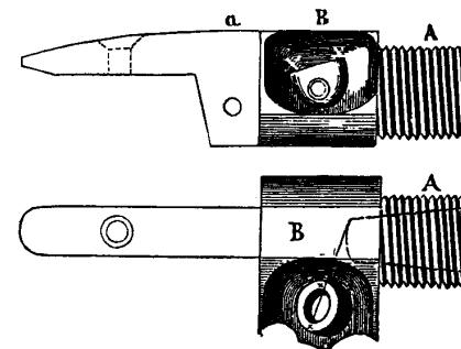
Fig. 12. Patentschwanzschraube. (Preußische von 1839.)
