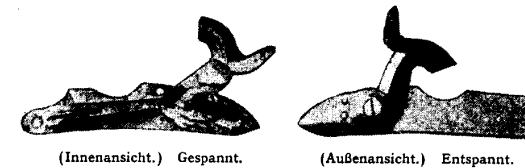
Fig. 11 a und b. Schloß des schweizerischen Infanteriegewehrs Modell 1842 (Perkussionskrappenschloß).
