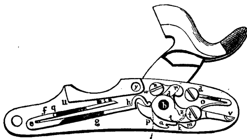
Fig. 11 c. Das Perkussionsschloß. (Preußisches von 1839.)
