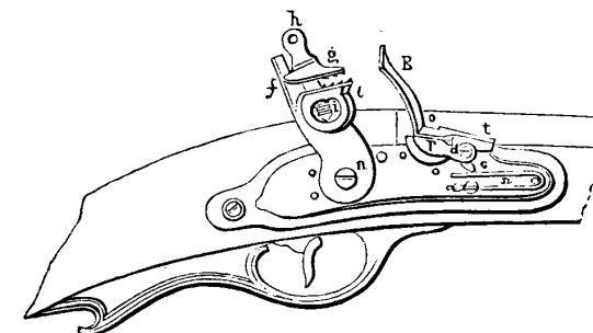
Fig. 6 a und b. Einrichtung des Steinschlusses.
