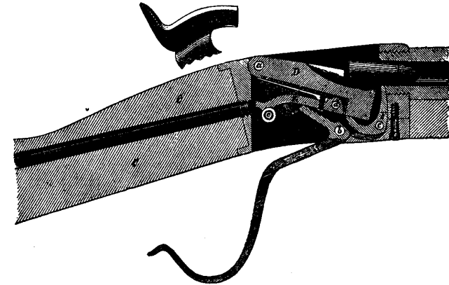
Fig. 40. Das System Peabody (Längsschnitt, geöffnet und geladen).
