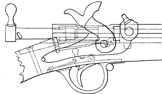
Fig. 35. Badische Jägerbüchse von 1863.
