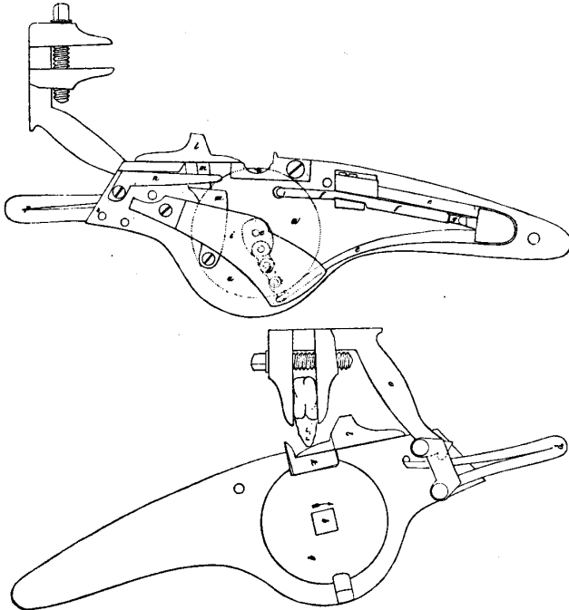
Fig. 3 a und b. Radschloß.
