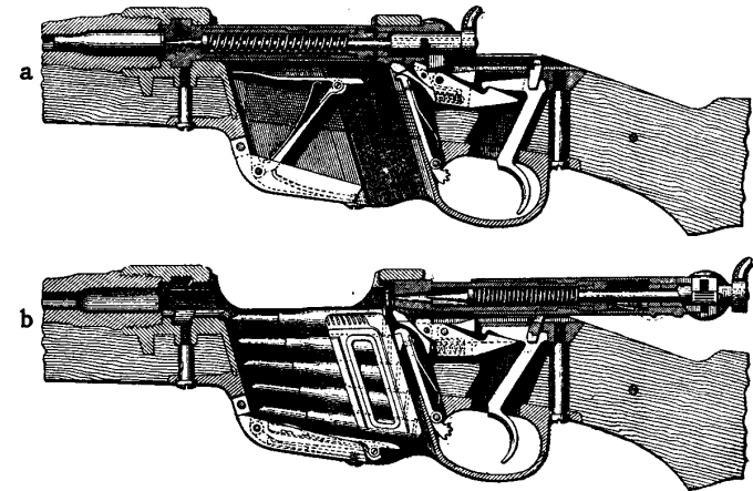
Fig. 66 a und b. Das System Mannlicher. Längsschnitt des Verschlusses, von links gesehen, des österreichisch-ungarischen Repetiergewehrs von 1895. a Verschuß geschlossen, abgefeuert, Magazin leer mit gehobenem Zubringer. b Verschuß geöffnet, gespannt, Magazin mit einem Rahmen (5 Patronen) gefüllt.
