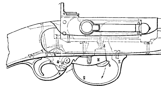
Fig. 33. Norwegisches Schützengewehr von 1848.
